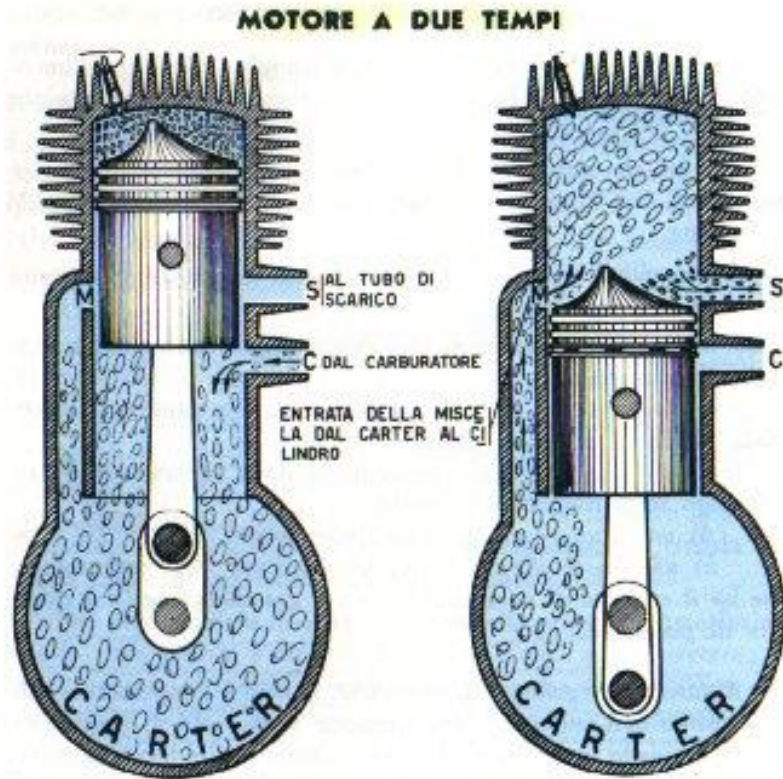
Fase di scoppio - Scarico del gas bruciato - Introduzione della miscela dal carter al cilindro
